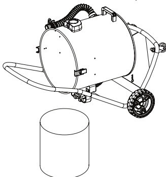
Fig. 15 – Retirando el material aspirado
