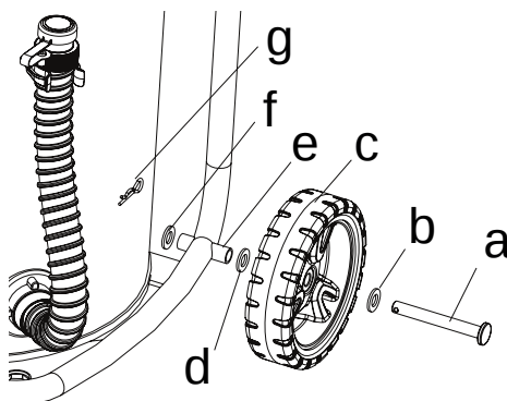
Fig. 4 – Instalação das rodas grandes
