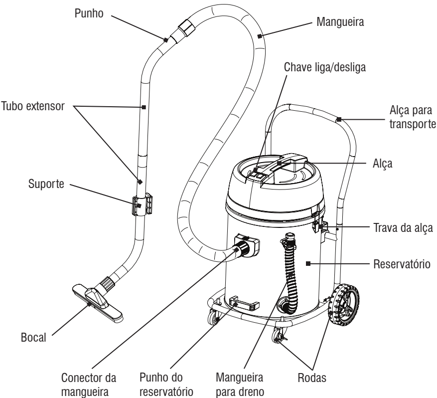
Fig. 1 – Componentes
