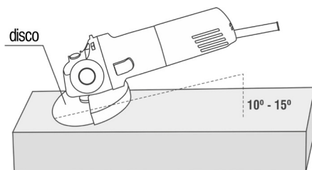
Figura 10 – Ângulo correto de esmerilhamento
