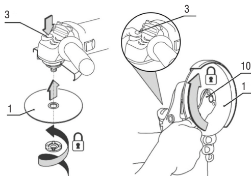
Figura 8 – Trocando o disco
