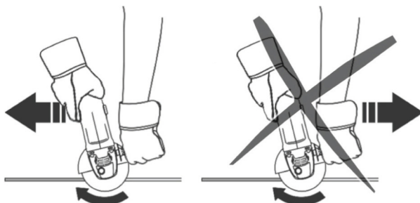
Figura 9 – Sentido de corte correto
