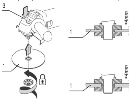
Figura 5 – Montaje del disco en la máquina
