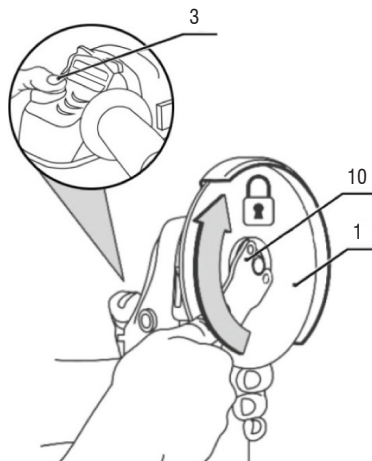
Figura 6 – Montagem do disco na máquina
