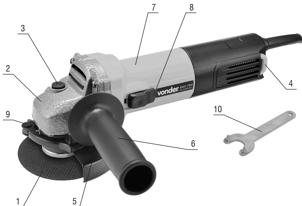
Figura 1 – Componentes de la Esmeriladora
