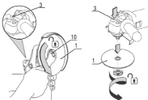
Figura 7 – Substitución del disco
