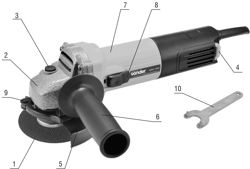
Figura 1 – Componentes da Esmerilhadeira
