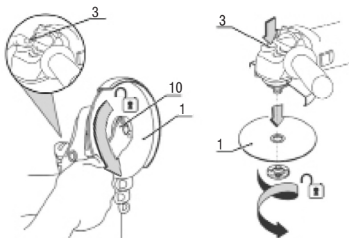
Figura 7 – Substituição do disco
