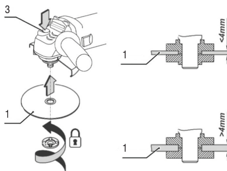
Figura 5 – Montagem do disco na máquina
