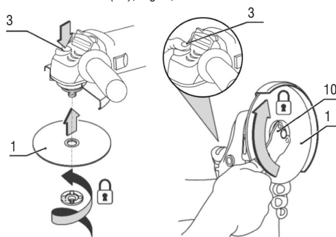
Figura 8 – Cambiando el disco
