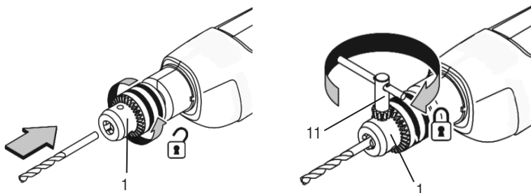
Figura 2 – Aperto da broca no mandril
