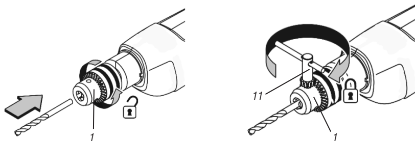
Figura 2 — Instalar la broca del mandril
