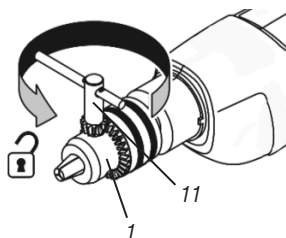
Figura 3 — Extraer la broca el mandril
