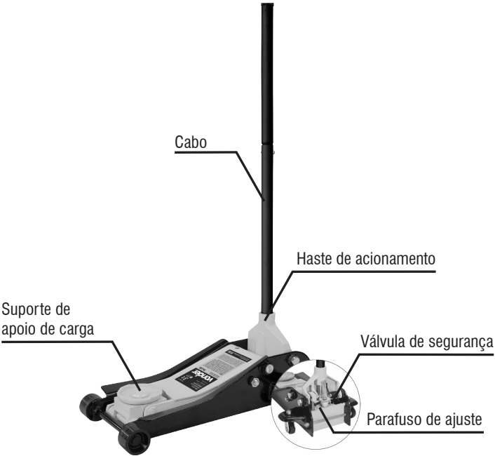
Figura 1 – Componentes
